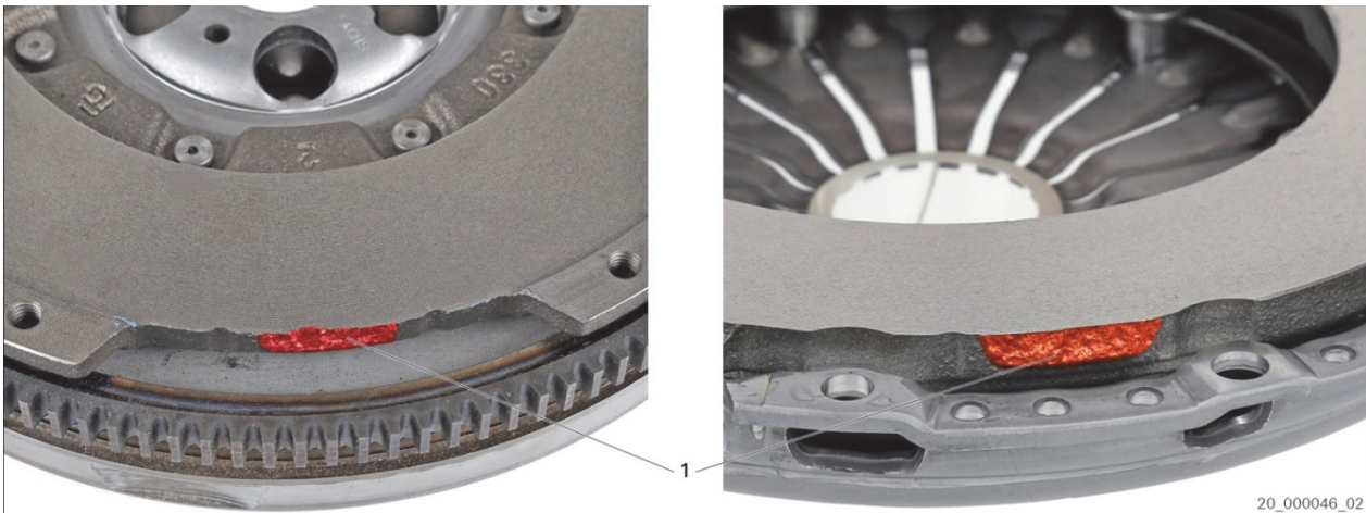
Рис. 1: Поверхность разрушения (пример)
