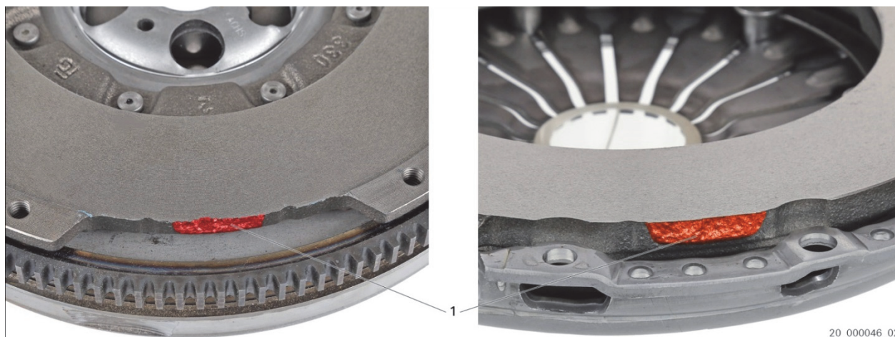
Rys. 1: Nieciągłość (przykład)
