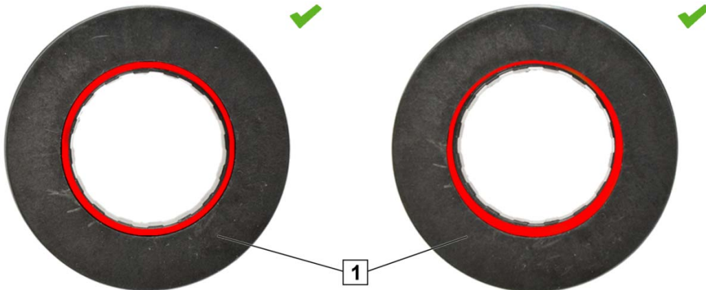
Fig. 1: Utløserlager med selv-sentrering. Lager sentrert og ikke sentrert (eksempel).
