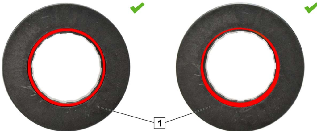
Afb. 1: Ontkoppelaar met zelfcentrerend. Lager gecentreerd en niet-gecentreerd (voorbeeld).
