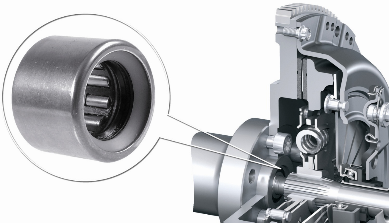
Fig. 1: kobling med styreleje
