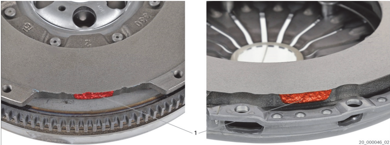
图示 1 : 破损边缘 ( 示例 )
