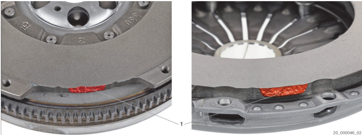
1pav.: Lūžimo briauna (pavyzdys)
