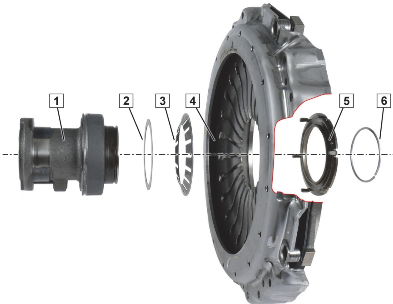
Obr. 1: Vypínací ústrojí spojky s pevným spojením. Pořadí montáže a uspořádání montážních dílů
