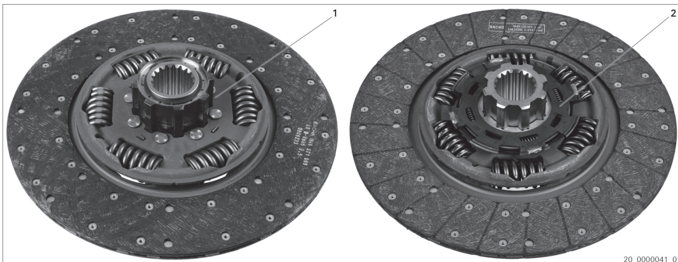
Рис. 1: Прежняя конструкция (пример)
