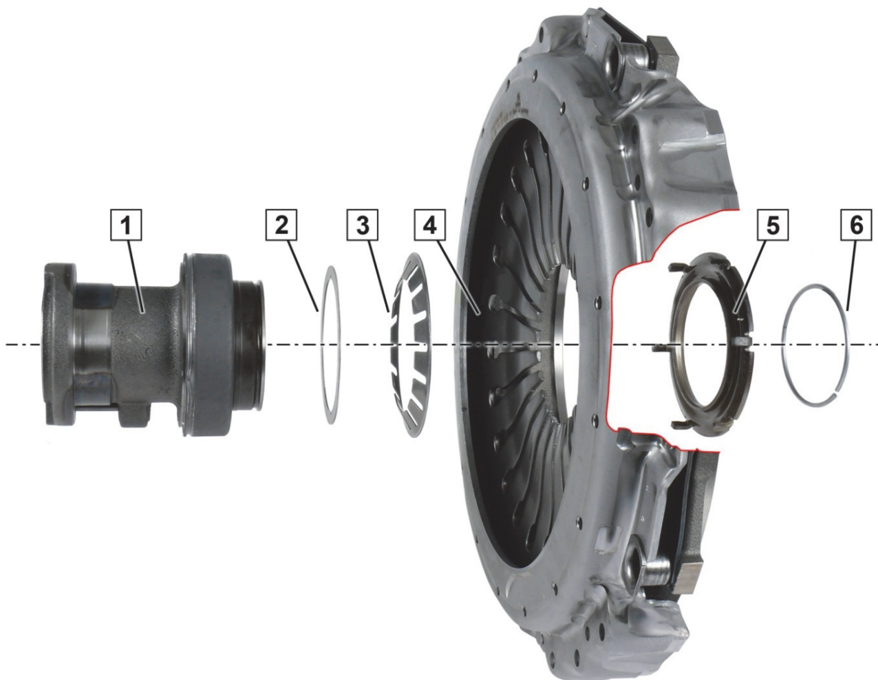
Рис. 1: Выжимной подшипник с неподвижным соединением. Последовательность установки и установочное положение деталей
