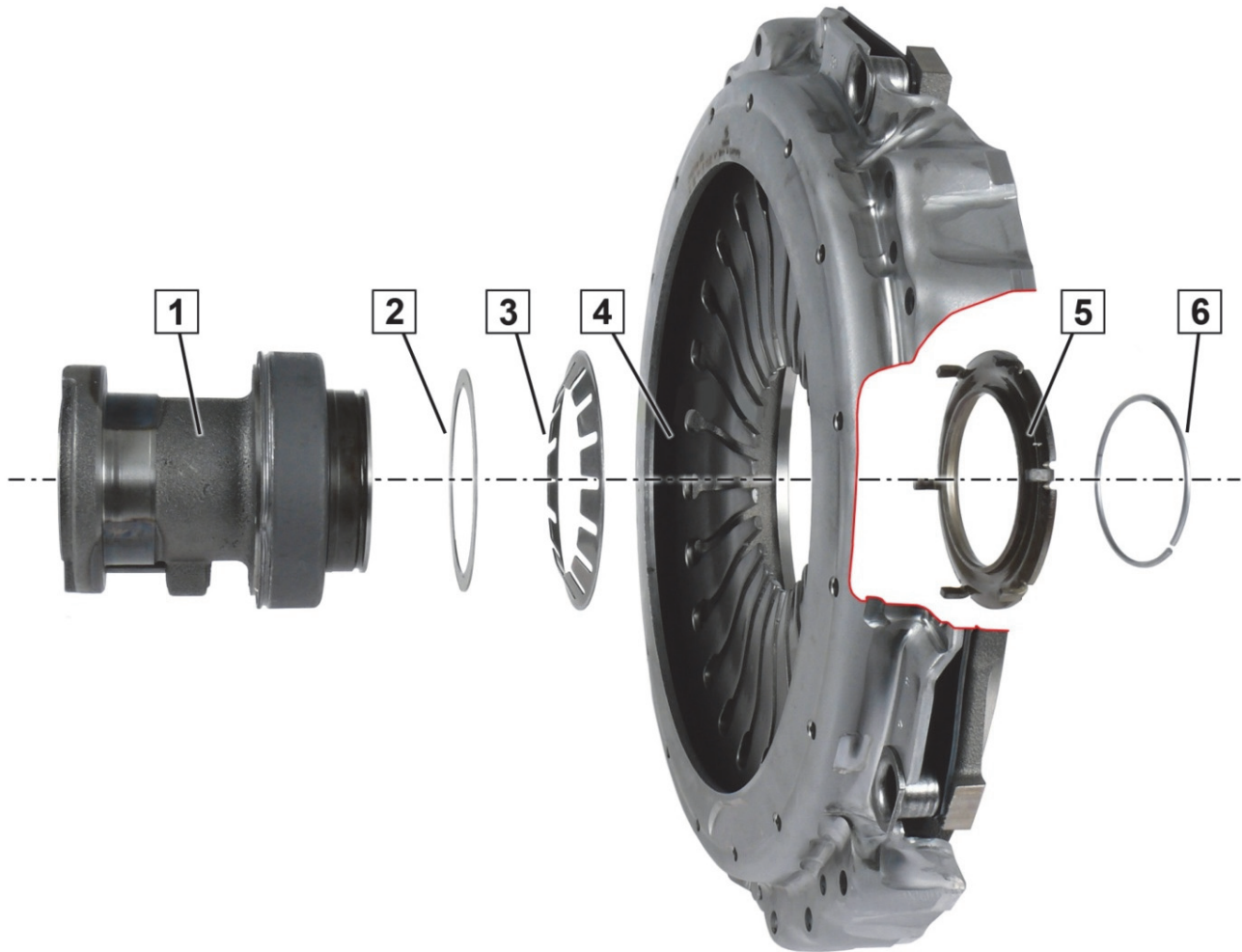
Fig. 1: Dispositivo de desembragem com ligação fixa. Sequência de montagem e orientação dos componentes
