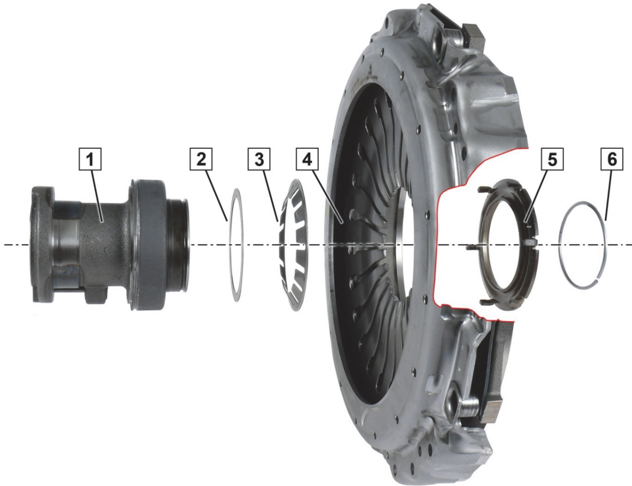
Afb. 1: Druklager met vaste verbinding. Montagevolgorde en afstelling van de onderdelen
