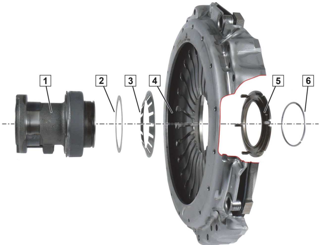
Fig. 1: Cuscinetto reggispinta con collegamento fisso. Sequenza di montaggio e allineamento dei componenti
