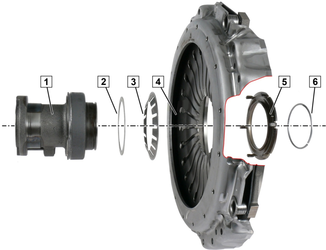
Fig. 1: Butée avec liaison fixe. Succession des opérations de montage et orientation des pièces
