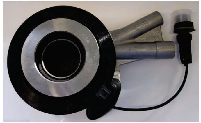
Abb. 4: 3182 600 101 mit Weg-Sensor
