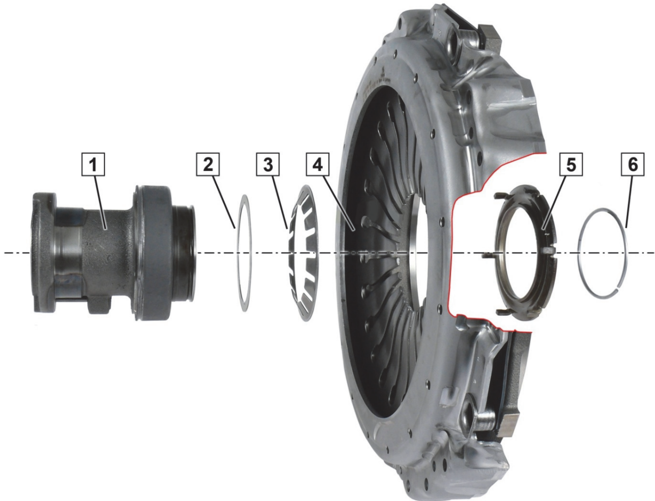
Fig. 1: udrykker med fast forbindelse. Monteringsrækkefølge og justering af komponenter
