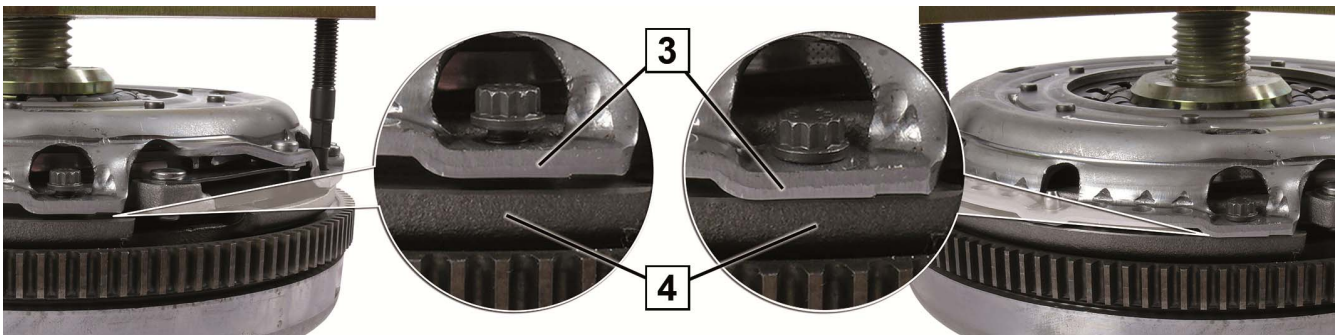
3. Ábra: A nyomólap előfeszítése
