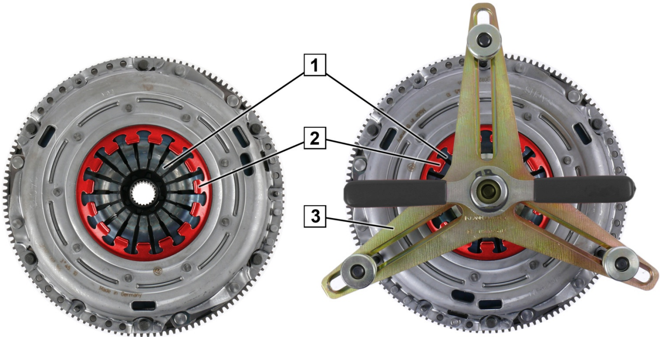
1. Ábra: Kiegészítő rugó
