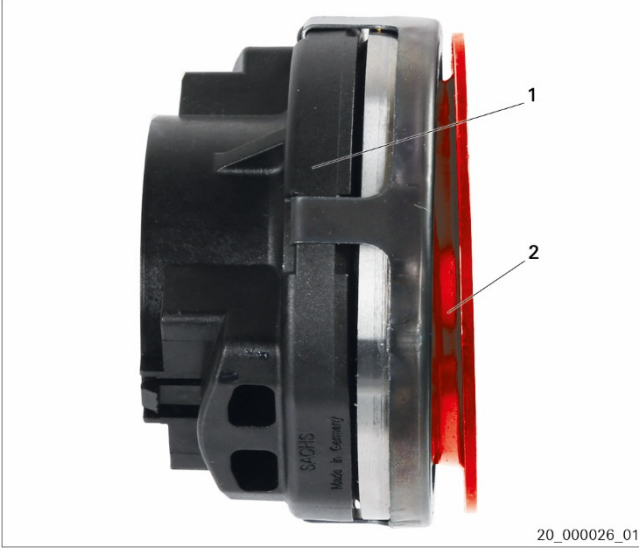
Resim 1: Balans ayarlı debriyaj rulmanı
