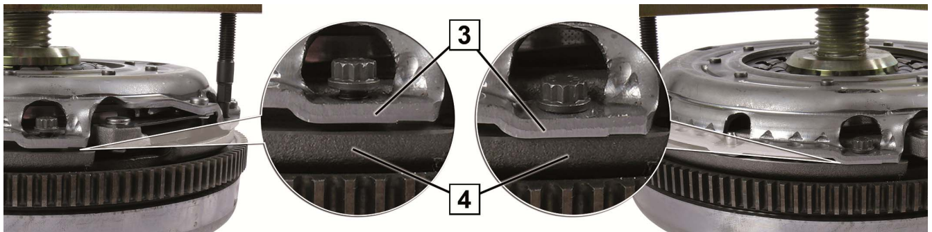
Sl. 3: Vpenjanje potisne plošče
