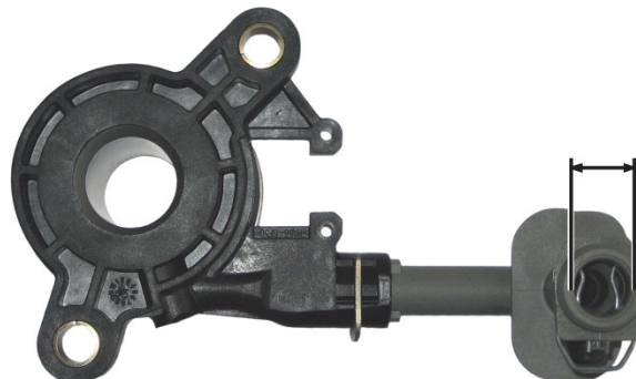
SI. 2: CSC 3182 600 129 → 3182 654 146 Premer hidravličnega priključka 13,3 mm
