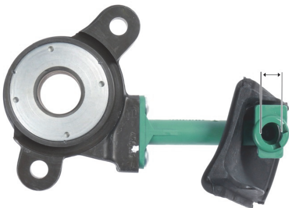
SI. 3: CSC 3182 600 120 Premer hidravličnega priključka 12,2 mm
