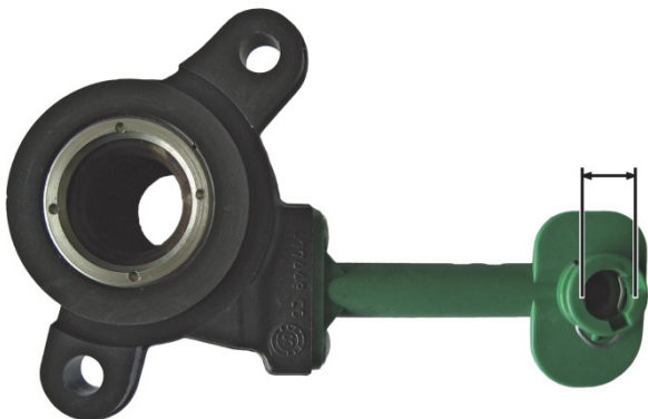
SI. 1: CSC 3182 600 121 → 3182 654 165 Premer hidravličnega priključka 11,7 mm
