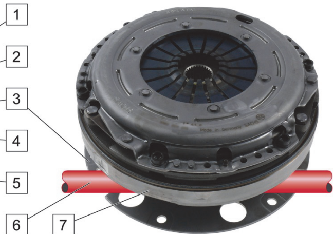
Fig. 2: Ambreiaj, volantă cu masă dublă (7) și planetară (6)
