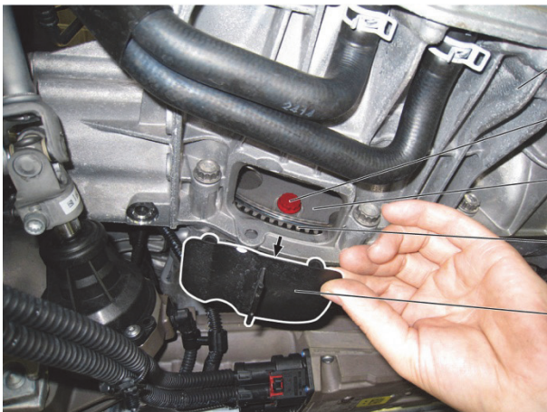
Fig. 1: Demontare capac (5)
