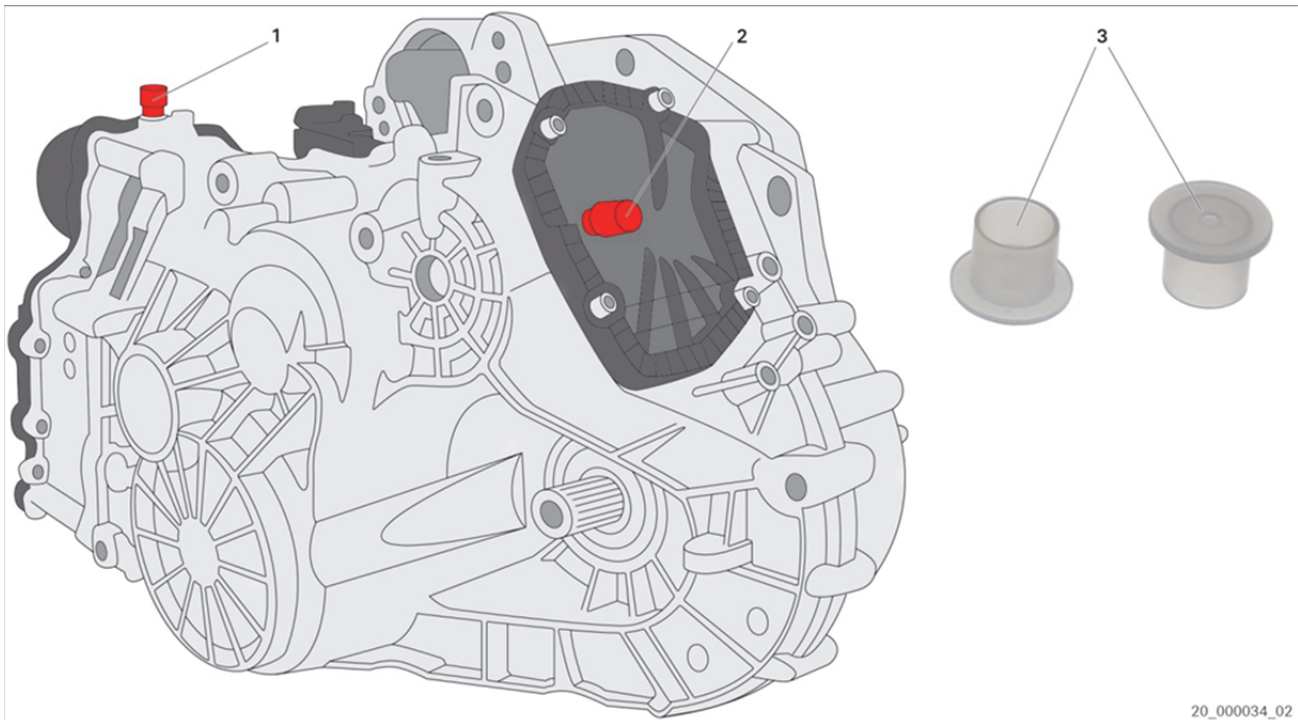
Sl. 1: Mjenjač s dvostrukom spojkom
