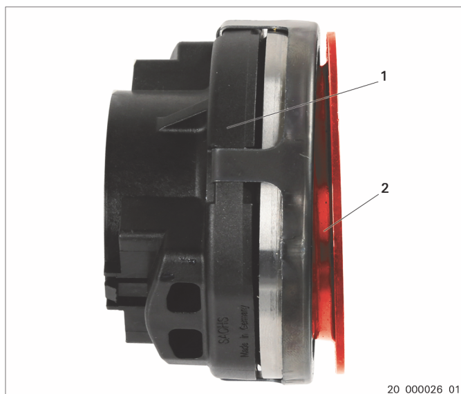
Fig. 1: Cuscinetto reggispinta con dispositivo di compensazione delle oscillazioni
