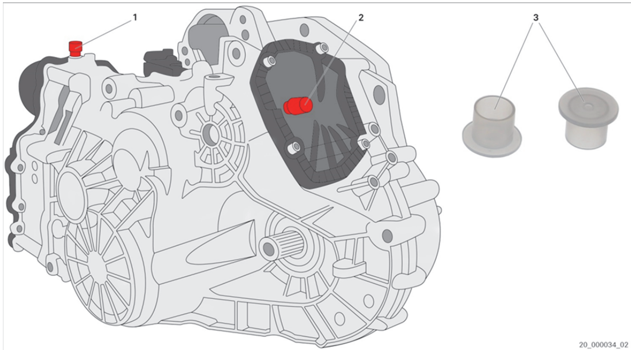
Εικ. 1: Κιβώτιο μετάδοσης διπλού συμπλέκτη
