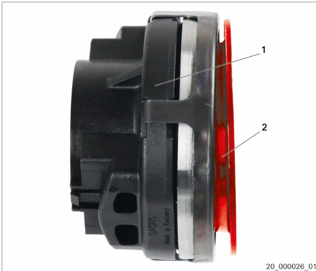
Fig. 1 : butée de débrayage avec dispositif compensateur de basculement
