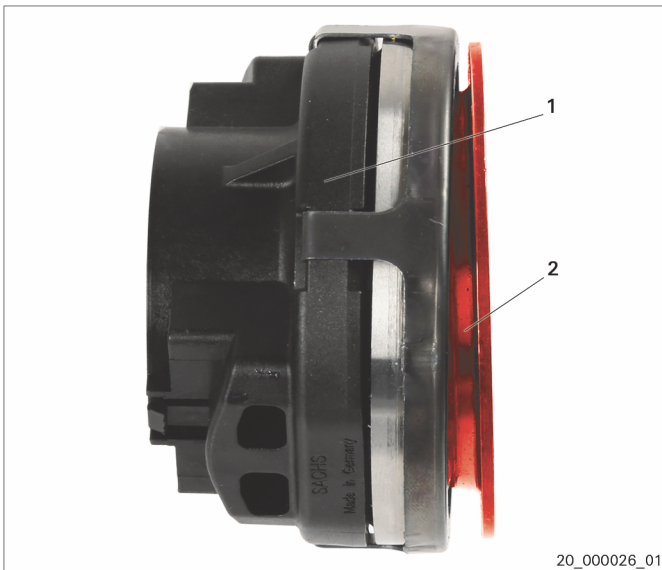
图示 1：带章动平衡功能的分离轴承
