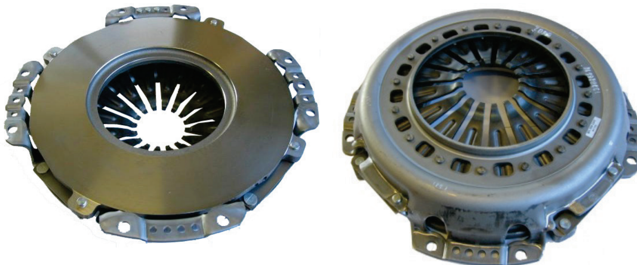
obr. 1: 330 mm jednoduchá spojka s membránovou pružinou
