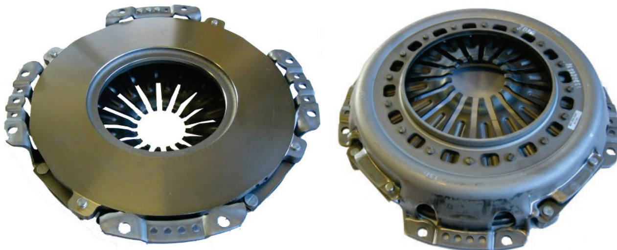
Fig. 1: 330 mm Embrague simple de muelle de diafragma
