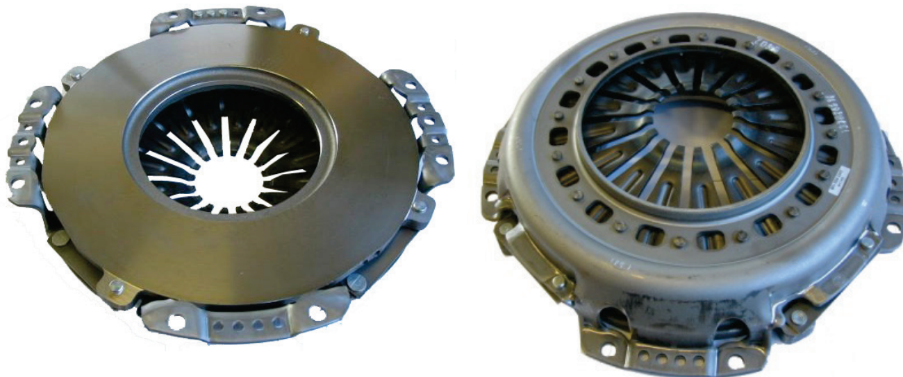
Obr. 1: 330 mm jednoduchá pružinová membránová spojka
