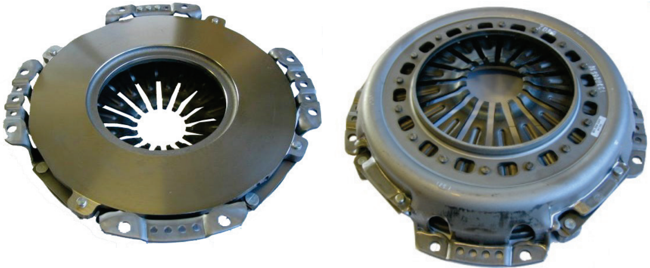
Bild 1: 330 mm enkel membranfjäderkoppling
