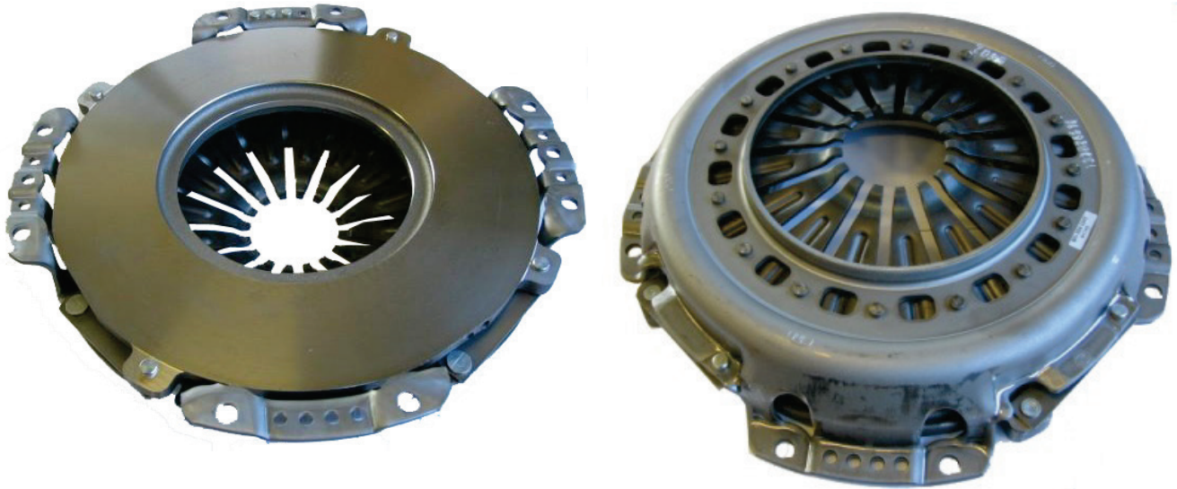
Illustr. 1: 330 mm enkelvoudige membraanveerkoppeling
