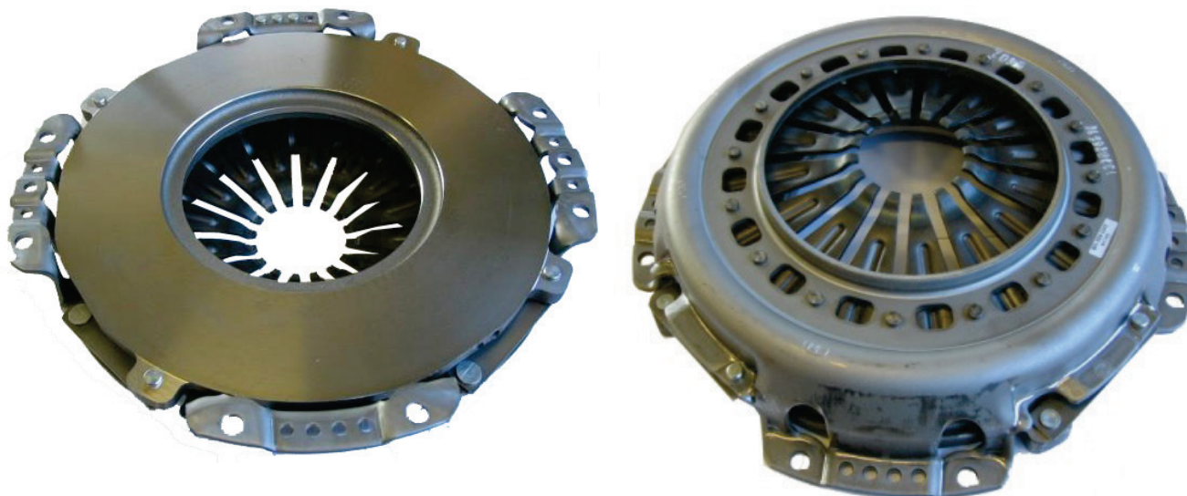
Sl. 1: jednostavna spojka s tanjurastom oprugom promjera 330 mm
