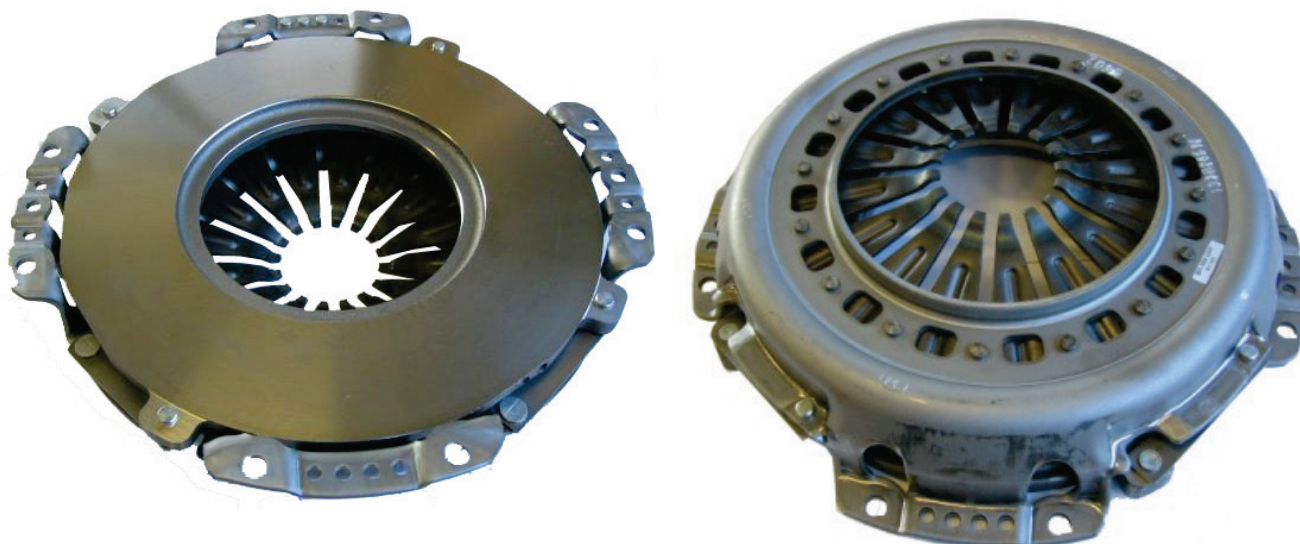
Fig. 1: frizione monodisco con molla a diaframma 330 mm
