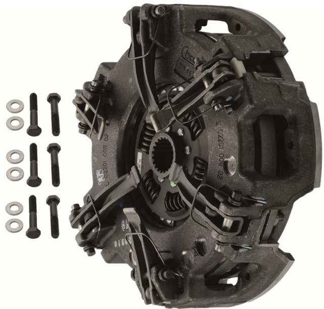
Fig. 2: frizione, modifica della costruzione
