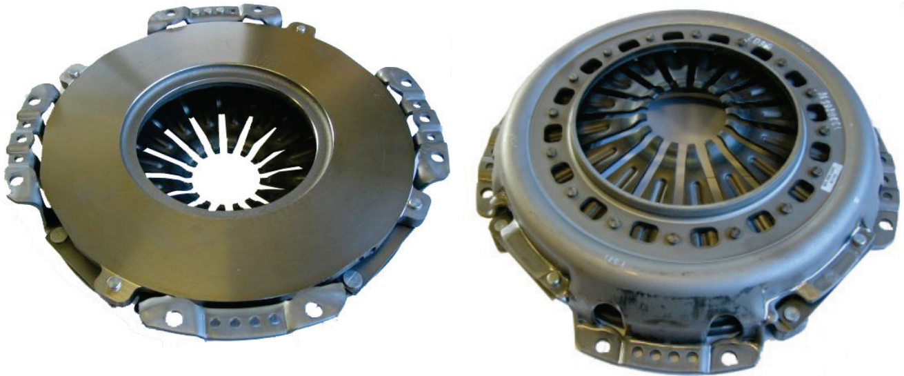
Εικ. 1: 330 mm Απλός συμπλέκτης ελατηριωτού διαφράγματος
