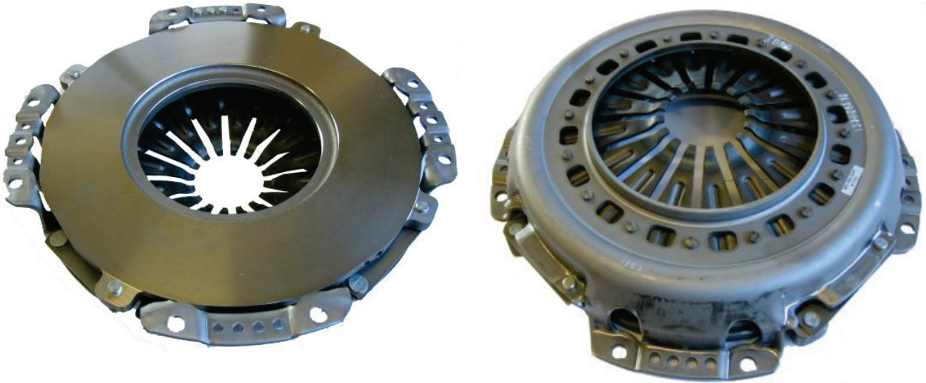
Kuva 1: 330 mm yksitasoinen kalvojouskytkin
