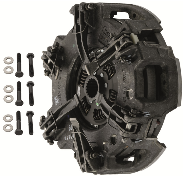
Kuva 2: Kytkin, rakenne muutettu
