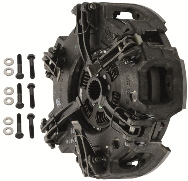
Abb. 2: Kupplung, Konstruktion geändert
