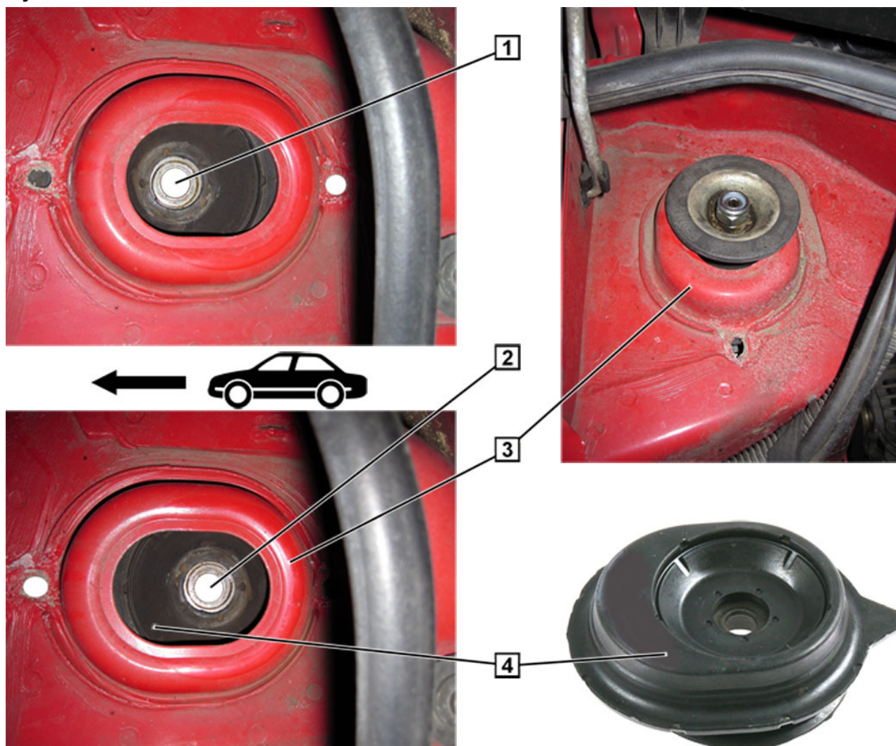
Obr. 1: Opěrné ložisko pružicí jednotky v různých montážních polohách
