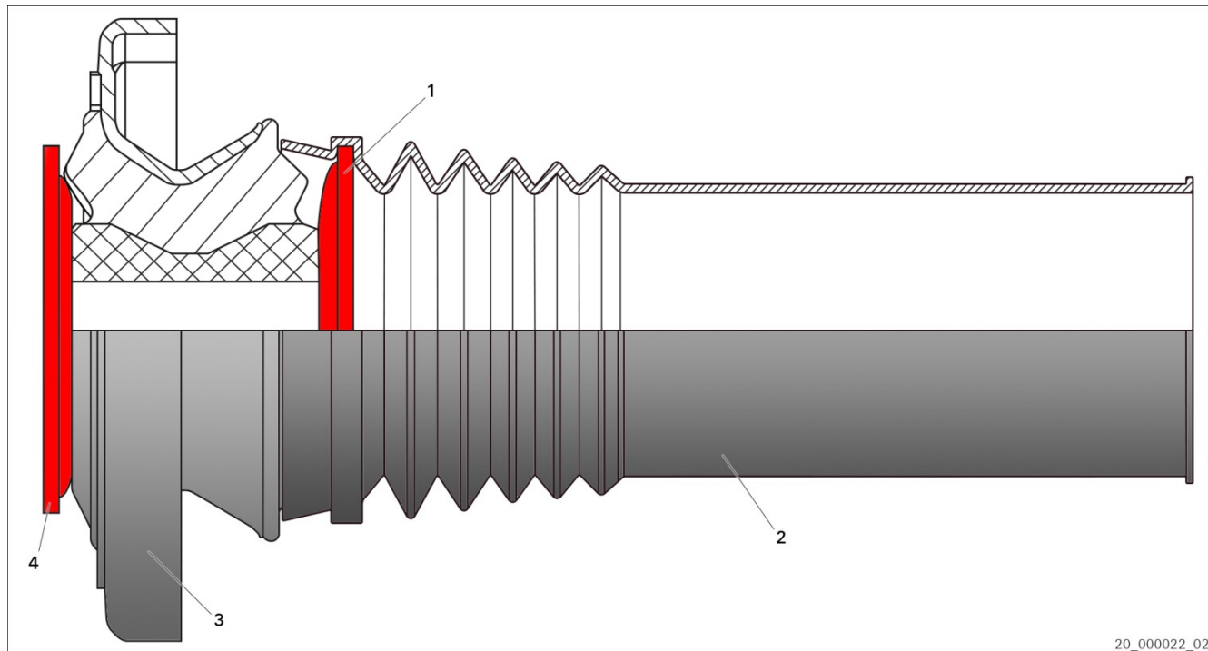
Εικ. 1: Έδρανο γονάτου ανάρτησης με ΚΙΤ σέρβις
