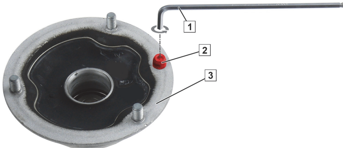
Fig. 1: Semelle pour jambe de force avec broche de positionnement
