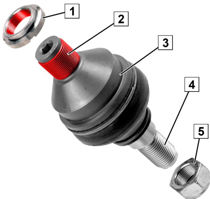
Sl. 1: Kuglasti zglob
