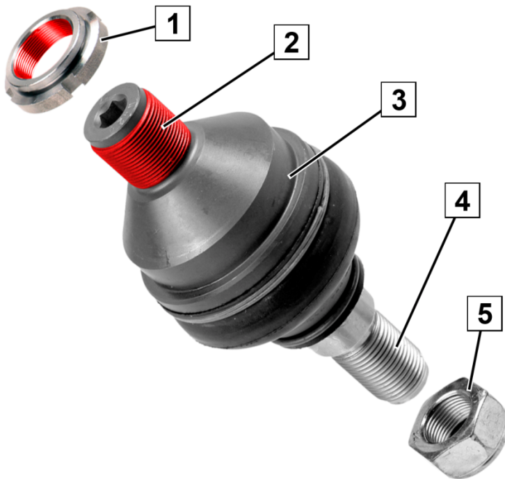
Fig. 1: Articolazione della sospensione
