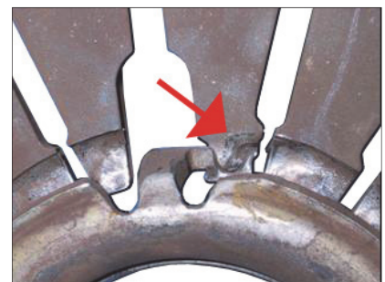
Fig. 5 : Usure excessive de la bague de débrayage et des languettes du ressort à diaphragme
