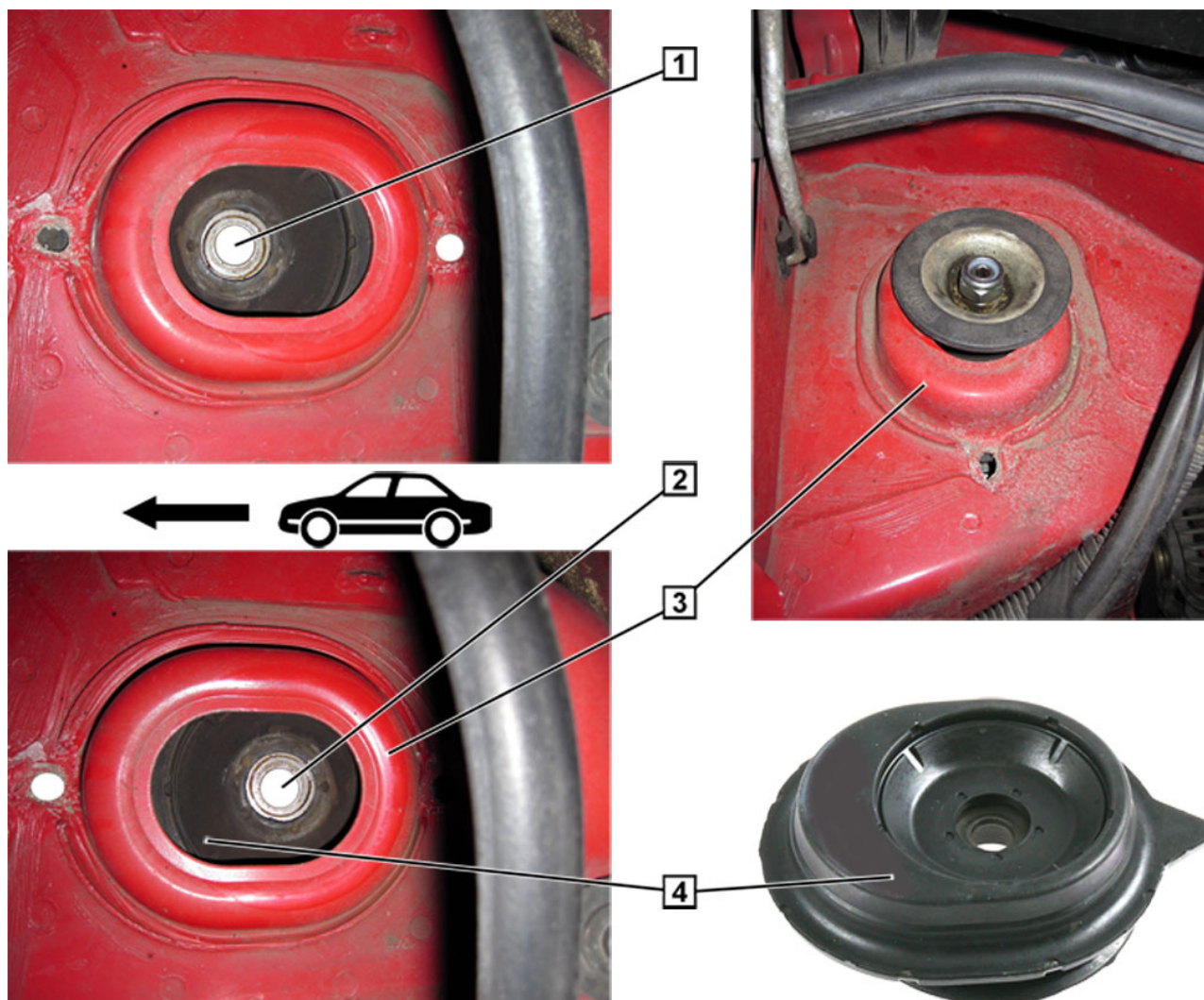
1. ábra: Toronycsapágó különböző beépítési helyzetekben
