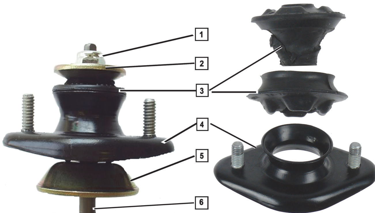
Obr. 1: Neporušené opěrné ložisko pružicí jednotky s montážními díly
