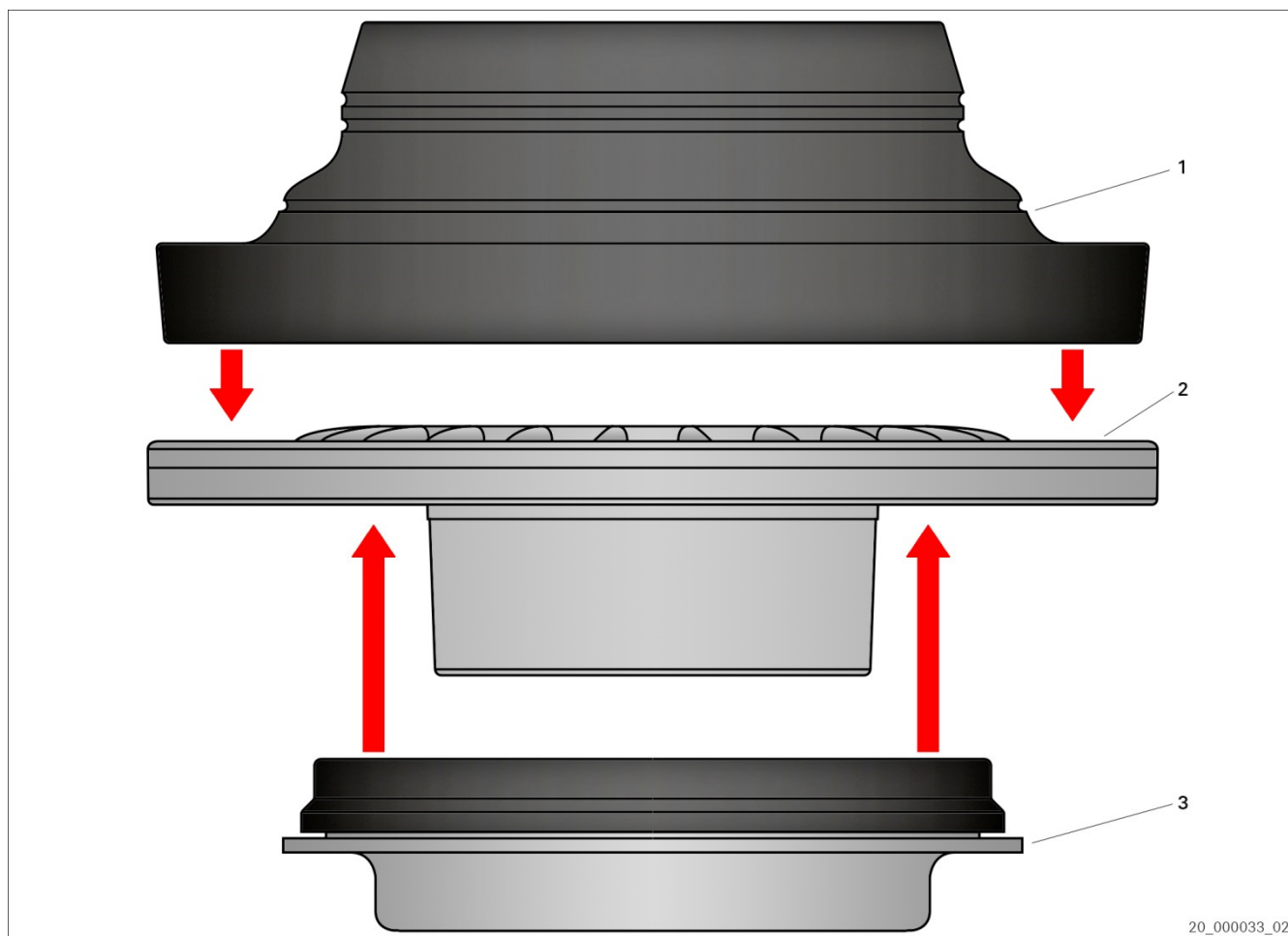
Fig. 1: Ensamblaje del soporte del puntal de suspensión (ejemplo)
