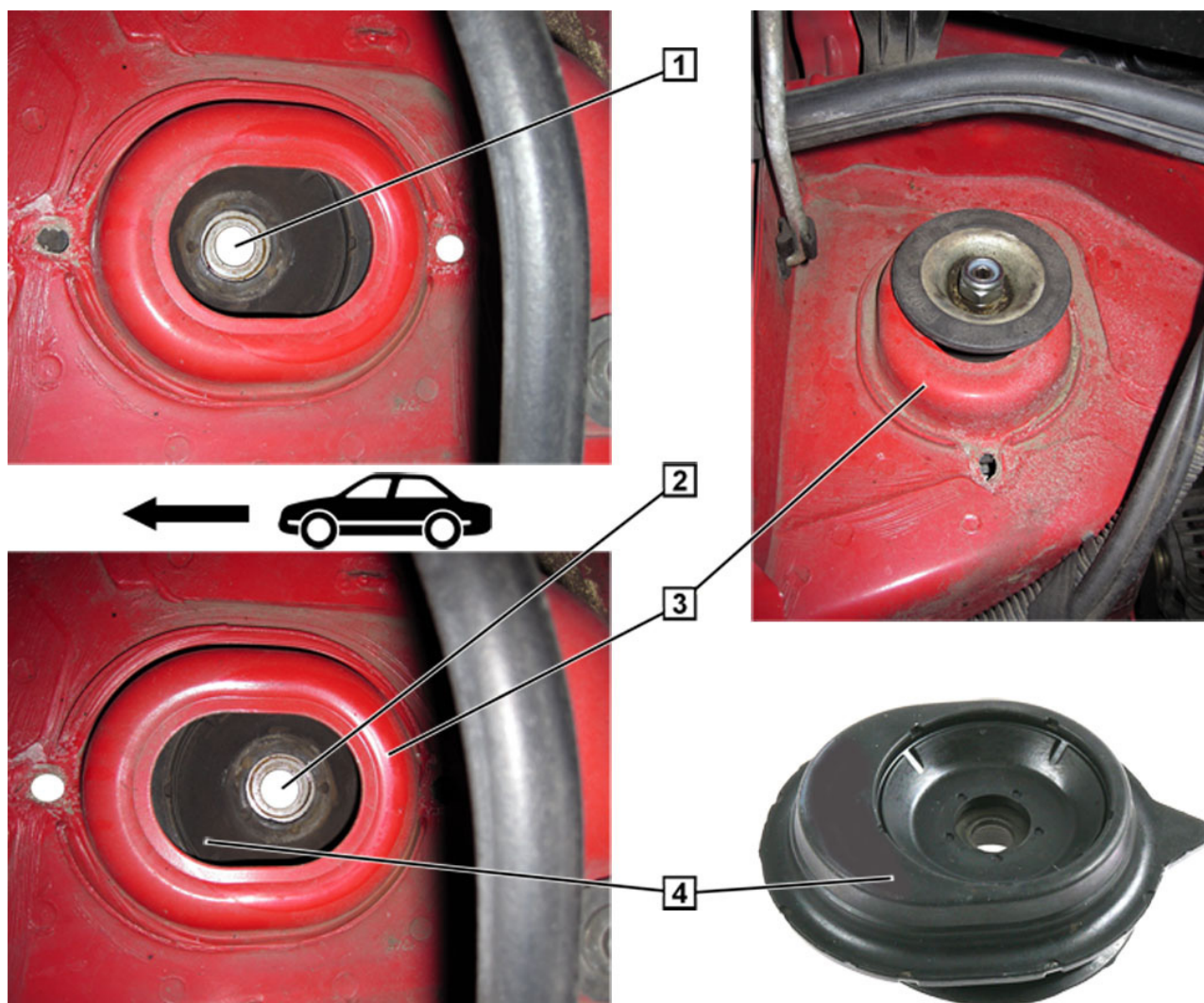
Sl. 1: Ležaj za oslanjanje u različitim položajima za ugradnju
