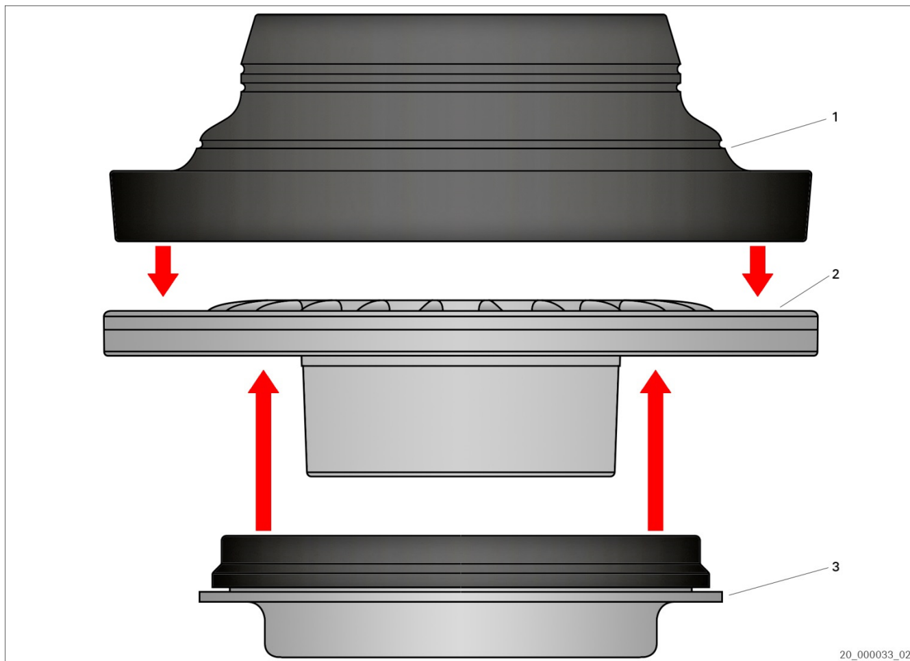
Fig. 1: Asamblarea crapodinei pentru piciorul arcului de suspensie (exemplu)
