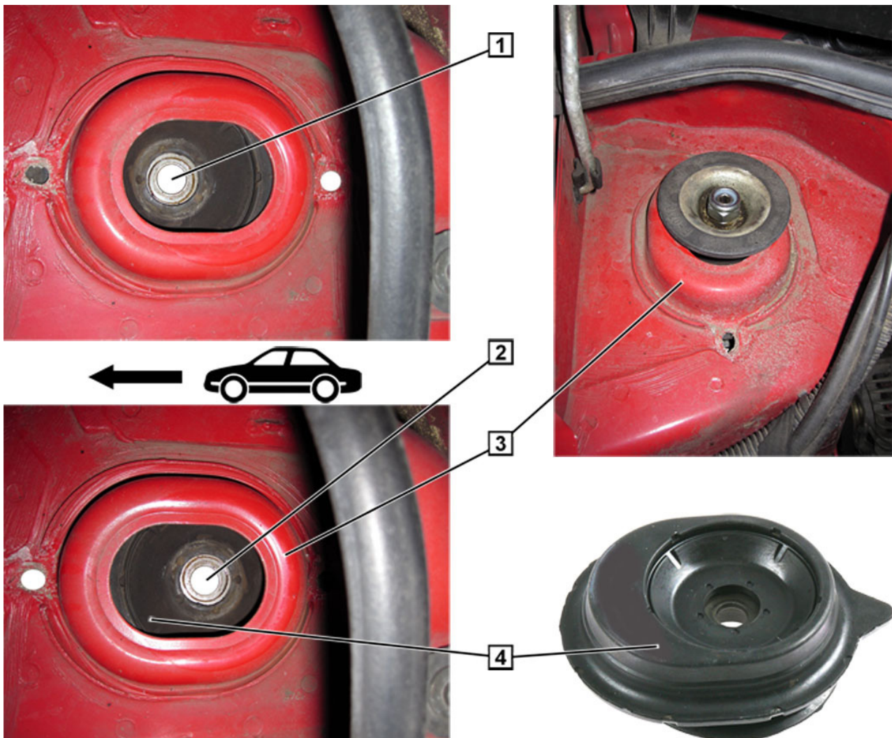
Illustr. 1: Veerpootsteunlager in verschillende inbouwstanden
